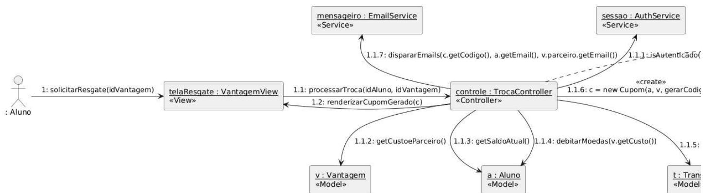
Diagrama de Comunicação: Fluxo Completo de Resgate de Vantagem (MVC)
